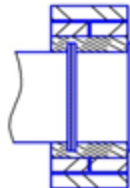
FSD-2...-H3-...-BH установка в преграде
