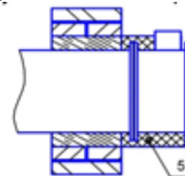
FSD-2...-H3-... установка вне преграды
