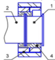
FSD-2...-H3-... установка в преграде
