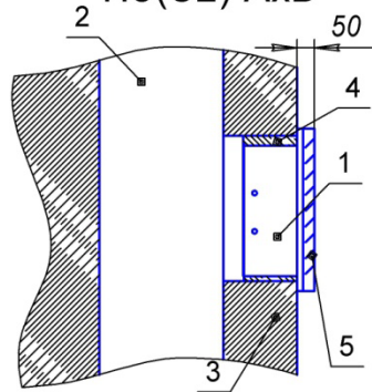
Рис. 4. Примеры схем установки клапана различных исполнений
