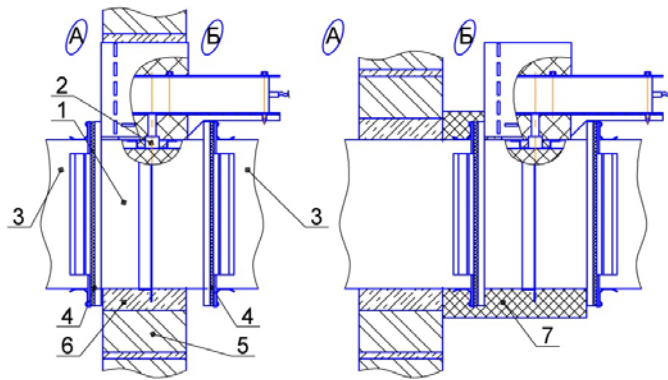
Рис. 4. Схемы установки клапана
