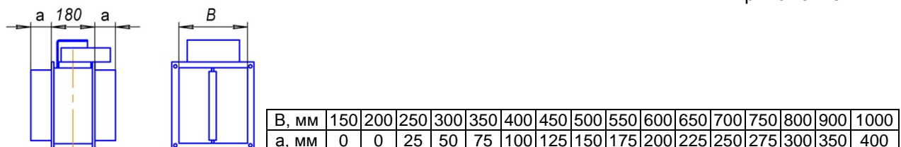
Рис.3. Размеры вылета заслонки в открытом положении за пределы корпуса клапана.
