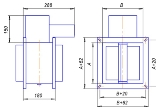
Рис.1. Установочные, габаритные и размеры внутреннего сечения клапана.
