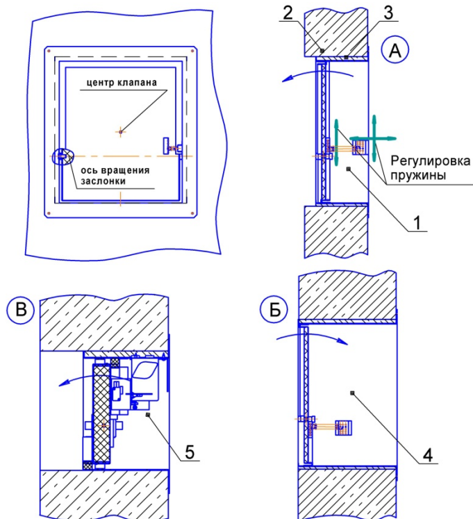
А - Тамбур-шлюз; Б – Шахта лифта; В – Сторона улицы. 1. Клапан исп. НЗ(КИД); 2. Строительная конструкция; 3. Цементно-песчаный раствор; 4. Клапан исп. НЗ(КИД)-Оп
