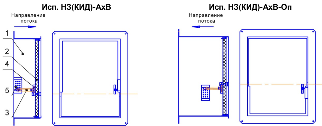
Рис. 2. Общие виды клапана.
